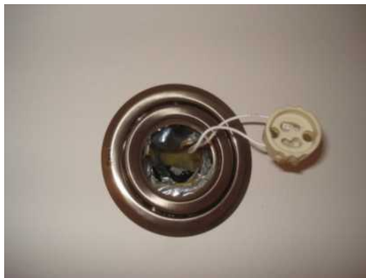
Poškození nevhodně umístěné parotěsné vrstvy při dodatečné montáži elektroinstalací
