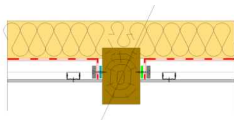
Napojení na dřevo butylovou oboustrannou páskou nebo Sunflex – pružným tmelem a přítlačnou lištou
