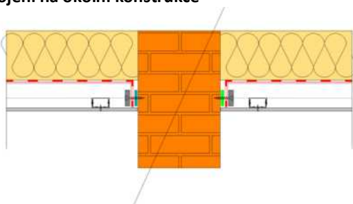
Napojení na zdivo butylovou oboustrannou páskou nebo Sunflex – pružným tmelem a přítlačnou lištou
